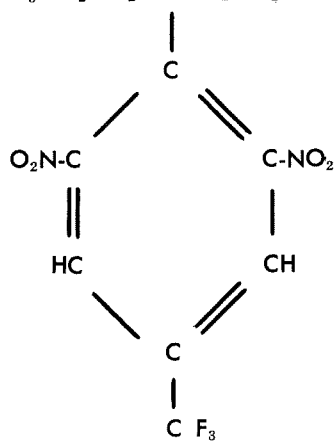
trifluralin
